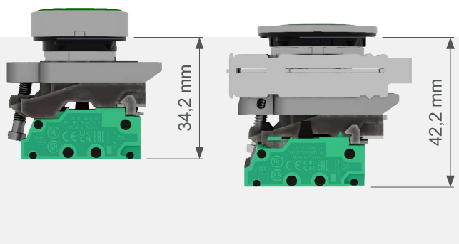
Standardní montáž
