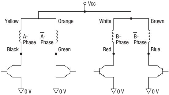
Fig. 4 Wiring
