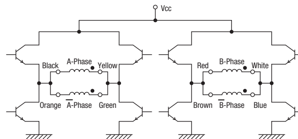
Fig. 8 Wiring
